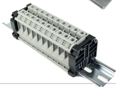
RAAK10N21-10 65 Amp, 600 Volt
