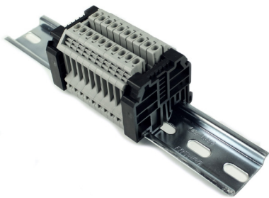
RAAK3N21-10 20 Amp, 600 Volt
