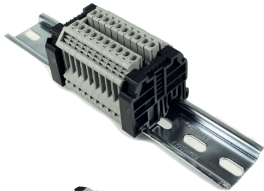
RAAK5N21-10 30 Amp, 600 Volt
