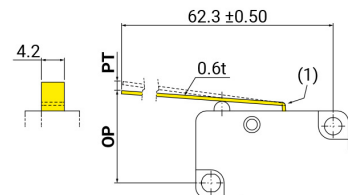
MFI.4STP
