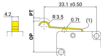
MFI.2STP
